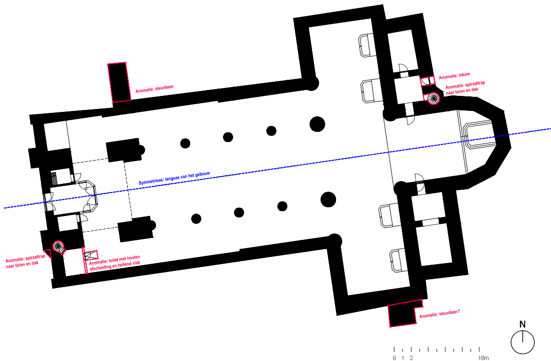
Afbeelding 60. Plattegrond met symmetrie en anomalieën van de O.L.V.-kerk.
