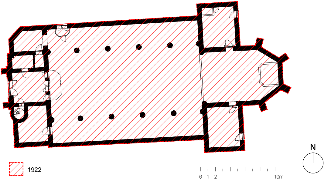
Afbeelding 10. Overzichtskaart met de verschillende bouwfases van de Heilig Kind Jezuskerk.
