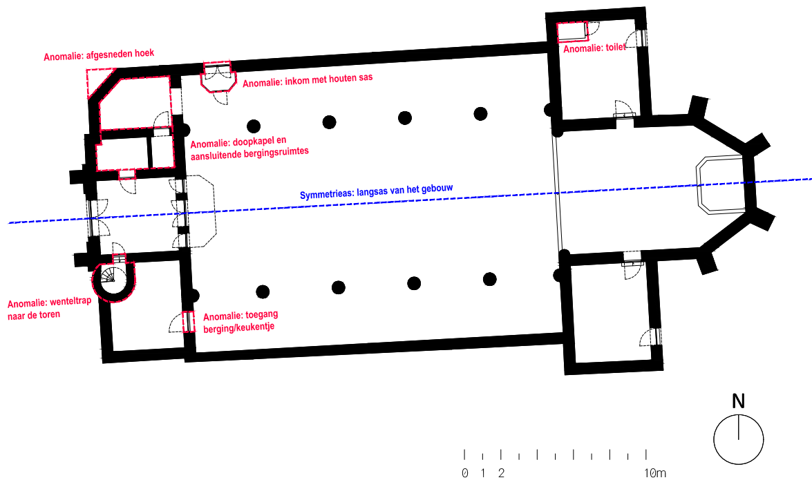
Afbeelding 61. Plattegrond met symmetrie en anomalieën van de Heilig Kind Jezuskerk in Kaggevinne.
