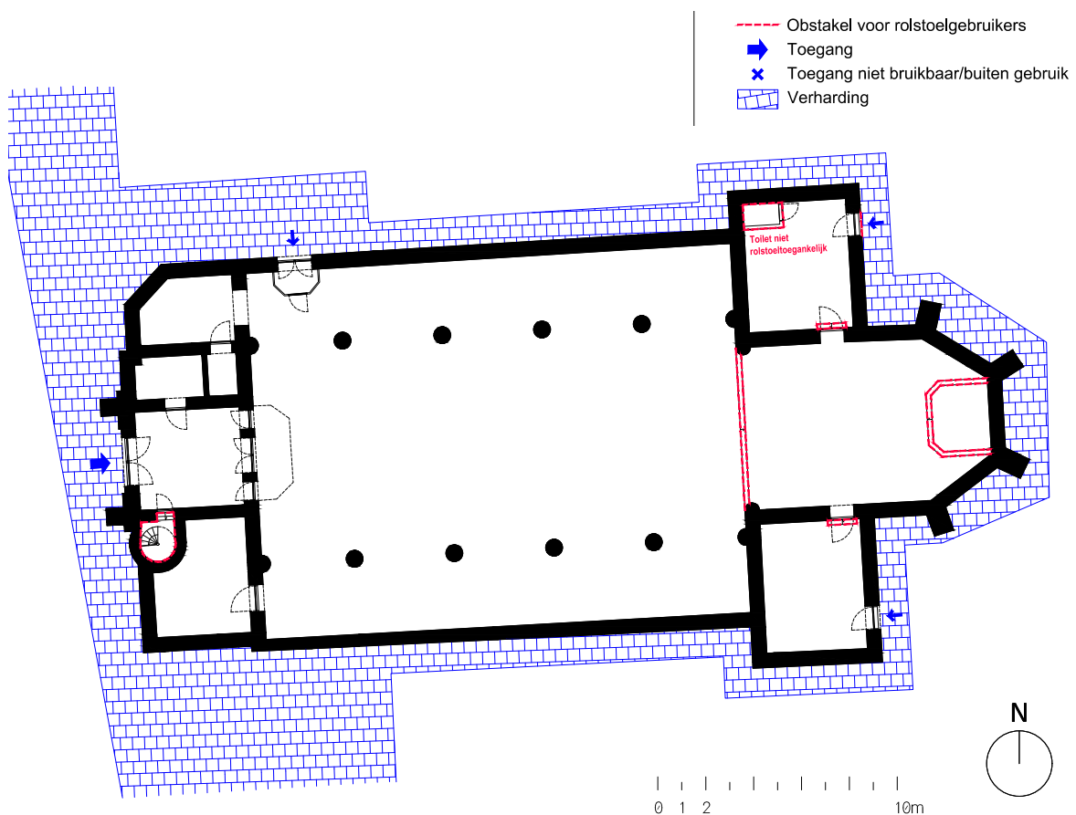
Afbeelding 62. Toegankelijkheidsplan van de Heilig Kind Jezuskerk van Kaggevinne.
